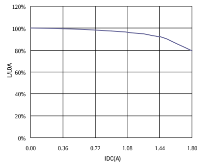
SR0805472KL□
