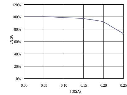
SR0805472KL□
